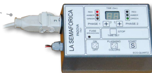
Particolare centralina
